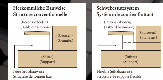
Bauweise der Resonanzbodenkonsole eines Klaviers Structure de la console de la table d'harmonie d'un piano droit
